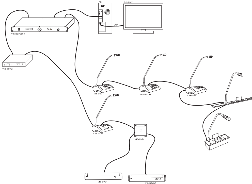
CLEACON-D Systemübersicht
