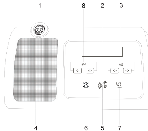
Präsidenten-Tischsprechstellen mit zweifacher Sprachwahlfunktion jeweils für linken und rechten Kopfhörer
