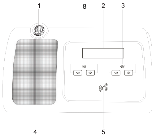
Delegierten-Tischsprechstellen mit zweifacher Sprachwahlfunktion jeweils für linken und rechten Kopfhörer
