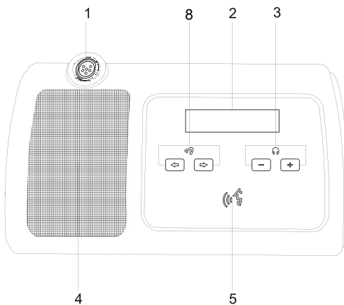
Delegierten-Tischsprechstellen mit Sprachwahlfunktion
