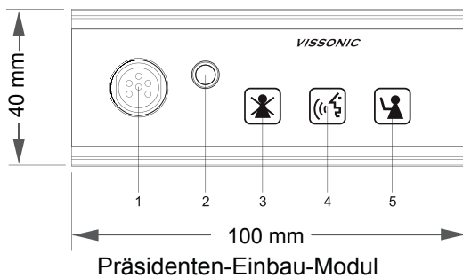
VIS-DCC-F
